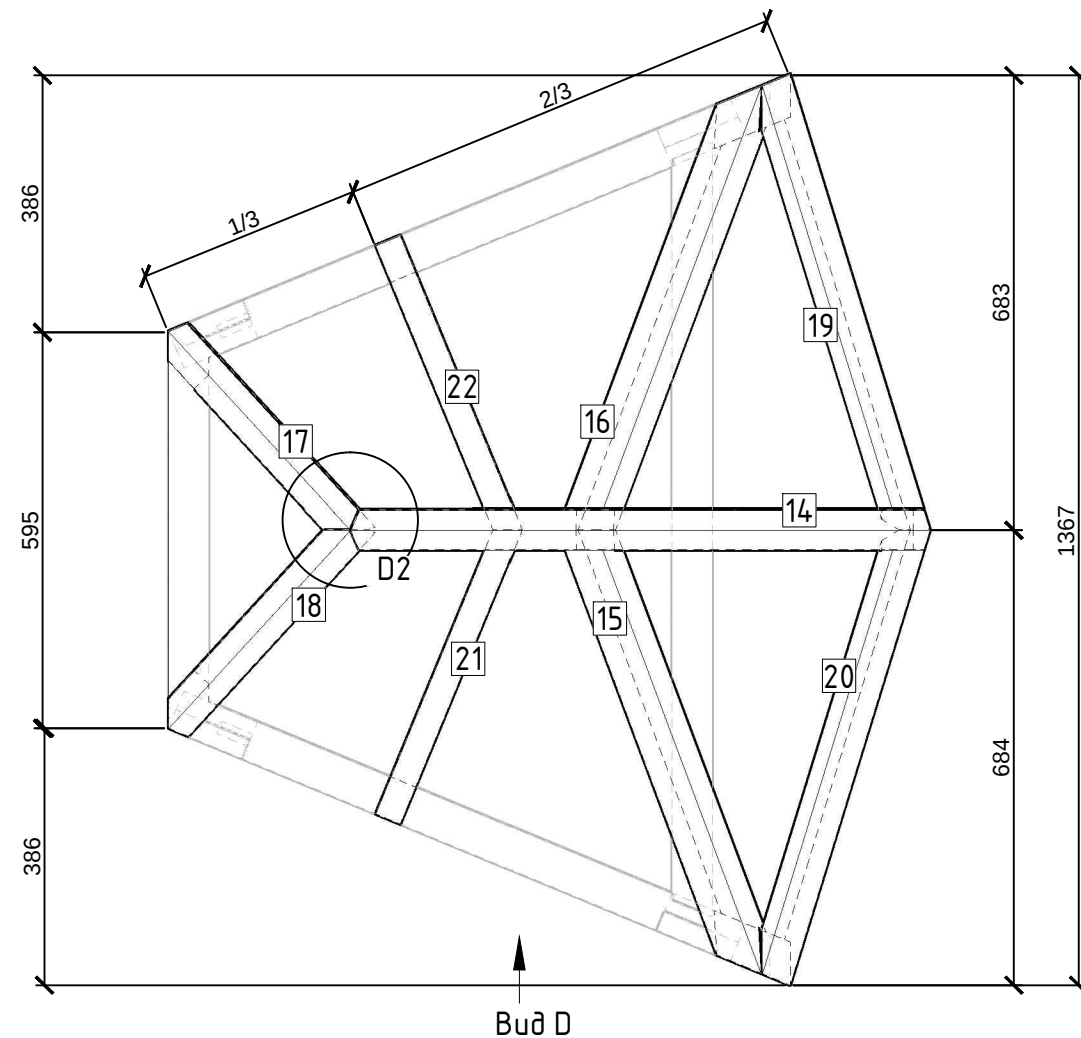
Вид сверху
